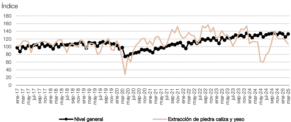
Gráfico 4.2.1 Extracción de piedra caliza y yeso respecto al nivel general del IPI minero, en números índice. Enero 2017-marzo 2025
