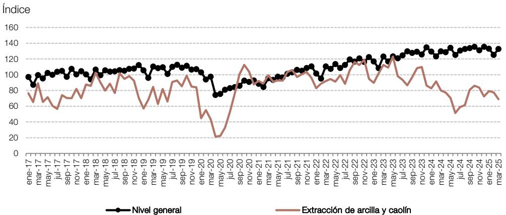
Gráfico 4.4.1 Extracción de arcilla y caolín respecto al nivel general del IPI minero, en números índice. Enero 2017-marzo 2025
